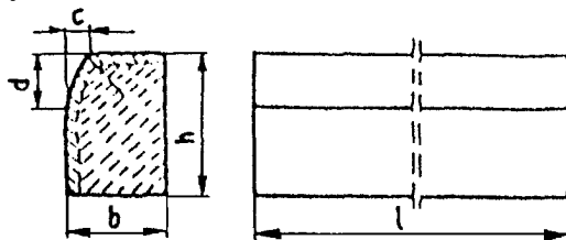
Rys. 1. Wymiarowanie krawężników
